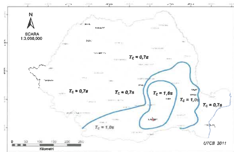
Figura 3.2 Zonarea teritoriului României în termeni de perioadă de control (c.c.). T_C a spectrului de răspuns
