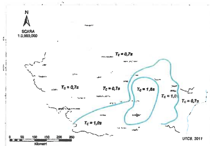
Zonarea Romaniei in termeni de perioada de control (colț), T_c a spectrului de raspun
