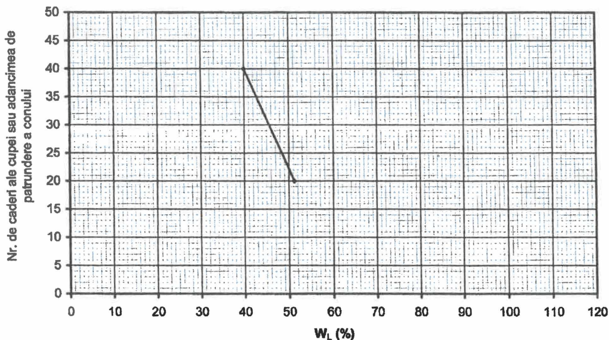
GRAFICUL LIMITEI SUPERIOARE DE PLASTICITATE
