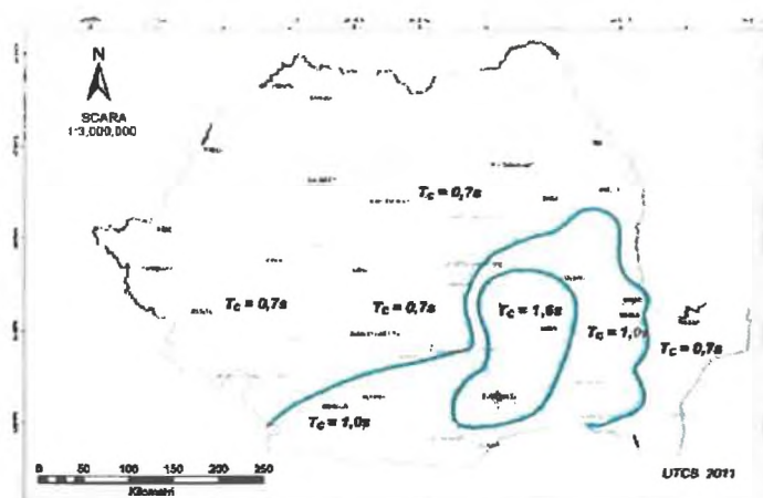
Figura A.2 Zonarea teritoriului României în termeni de perioada de control (ciclul). T_c a spectrului de răspuns
