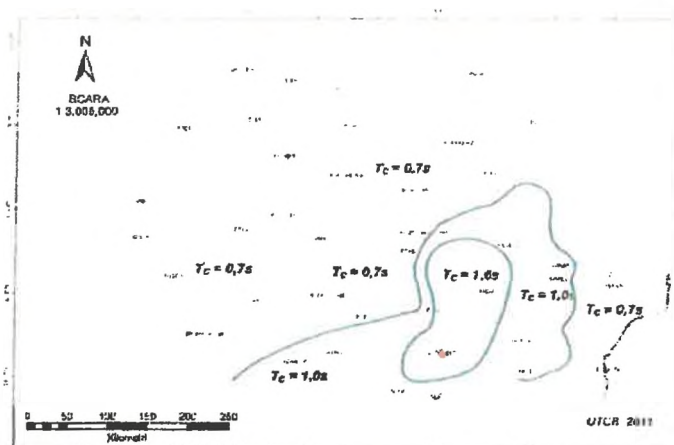
Figura 3.2 Zonarea teritoriului Râmnicu Vâlcea în termeni de perioadă de control (cod). T_c a spectrului de răspuns
