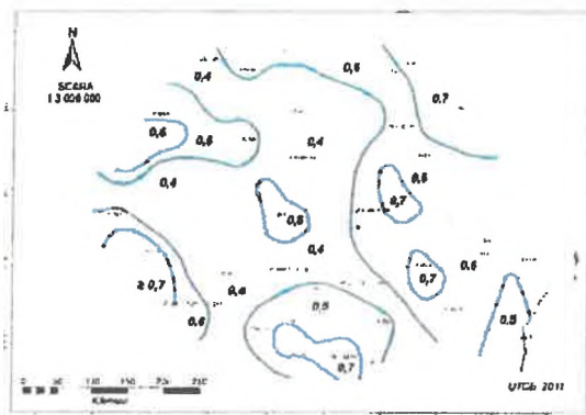
Figura 2.1 Zonarea valorilor de referinta ale presiunii dinamice a vântului, p în kPa, având = 50 ani. NOTA. Pentru altitudini peste 1000m valorile presiunii dinamice a vântului se corectează cu relația (A.1) din Anex
