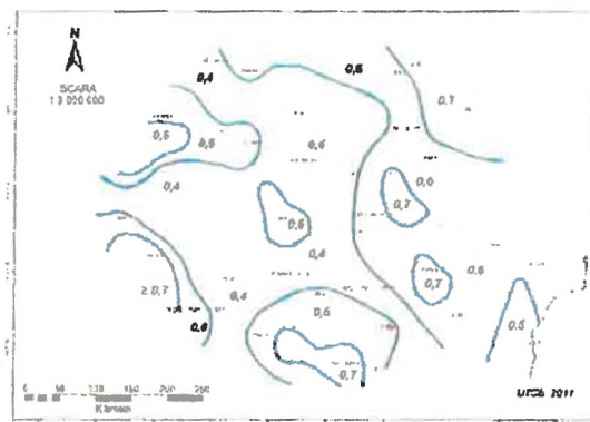
Figura 2.1 Zonarea valorilor de referinta ale presiunii dinamice a vântului, s în kPa, având = 50 ani NOTA. Pentru altitudini peste 1000m valorile presiunii dinamice a vântului se corecteaza cu relatia (A.1) din Anex
