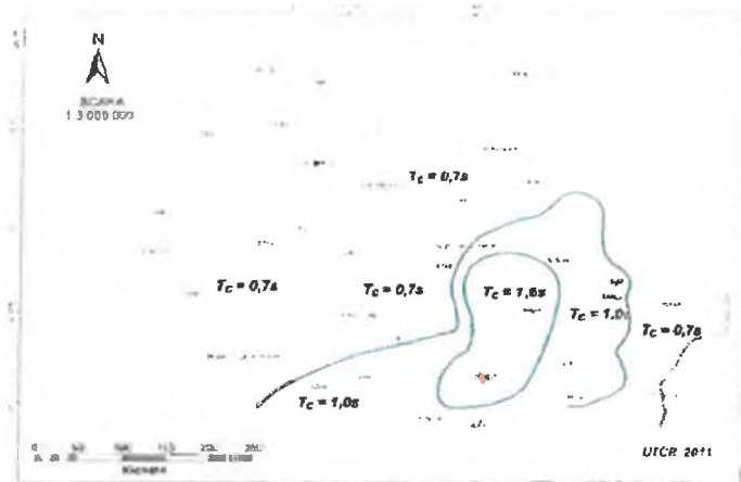
Figura A.2 Distribuția riscului seismic în România în termeni de perioadă de control (ciclul T_c ) a spectrului de răspuns
