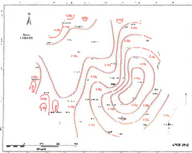
Figura XI România- Zonarea valorilor de vârf ale accelerației terenului pentru proiectare cu IMR = 225 ani și 20% probabilitate de depășire în 50 de ani
