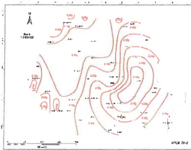
Figura 3.1 România - Zonarea valorilor de vârf ale accelerației terenului pentru proiectare a_g cu \text{IMR} = 225 ani și 2\sigma , probabilitate de depășire în 50 de ani
