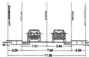
PROFIL B-B' DRUM PROPUȘ
