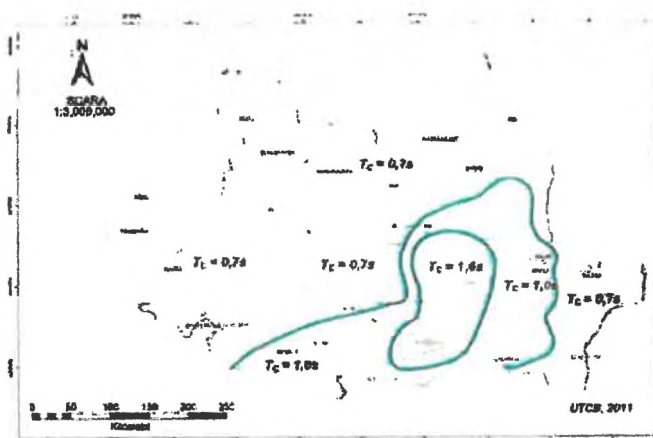
Figura 3.2 Zonarea teritoriului României în funcție de perioada de control (Tc), Tc - a spectrului de răspuns
