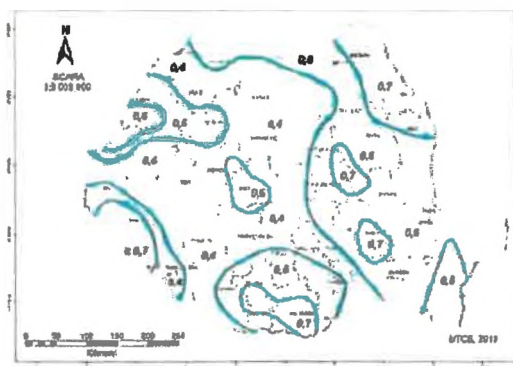
Figura 2.1 Zonarea valorilor de referinta ale presiunii dinamice a vântului, p în kPa, având = 50 ani NOTA. Pentru altitudini peste 1000m valorile presiunii dinamice a vântului se corectează cu relația (A.1) din Anex
