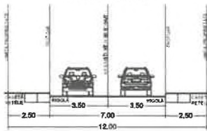
PROFIL A-A' MODERNIZAT EXISTENT ȘI PROPUȘ STRADA BICAZ
