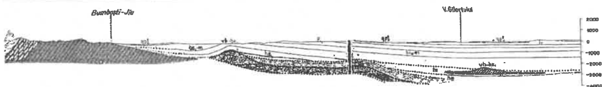
Figura 5. Secțiune geologică prin zona de amplasament
