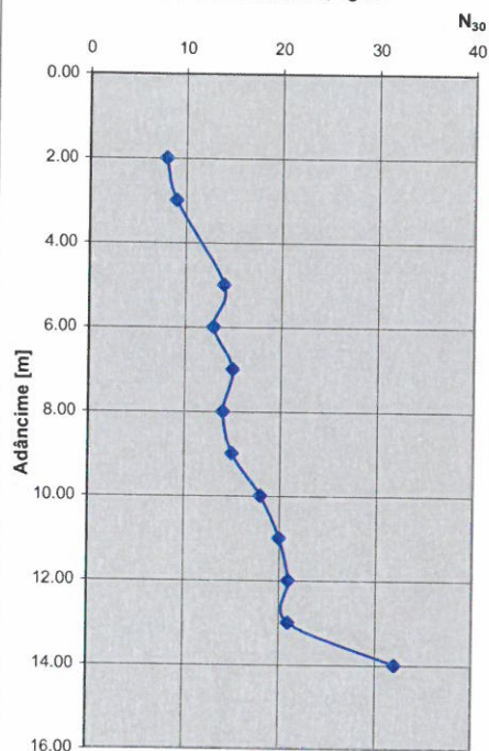
Rezultate SPT Scoala Gimnaziala nr. 8, Tg-Jiu
