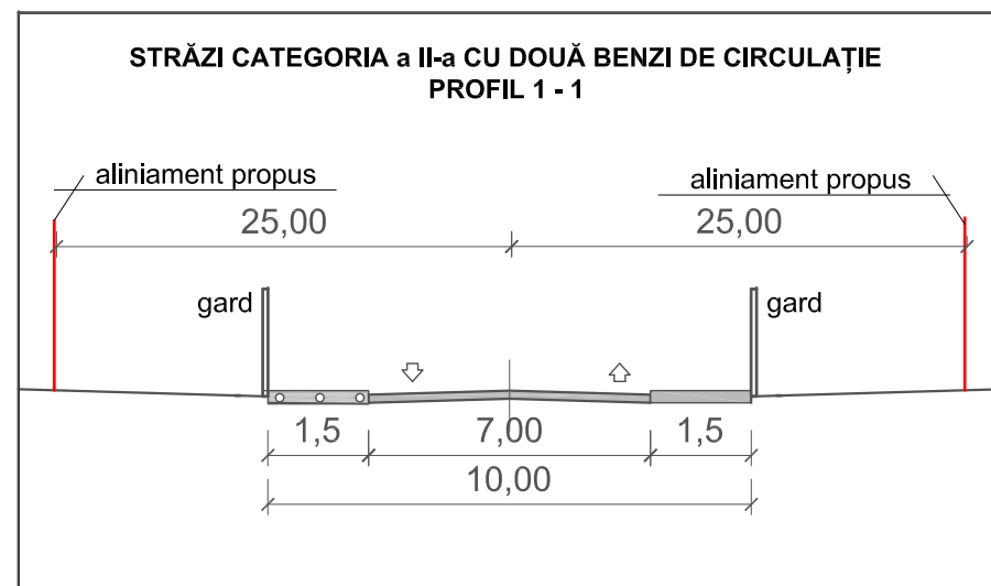
PROFIL STRADALE PROPUSE
